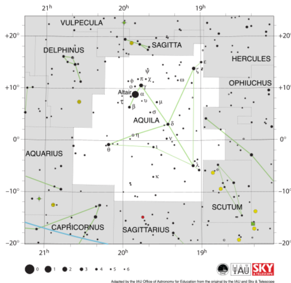
Figure 1: Carte du ciel de la région de BH3
