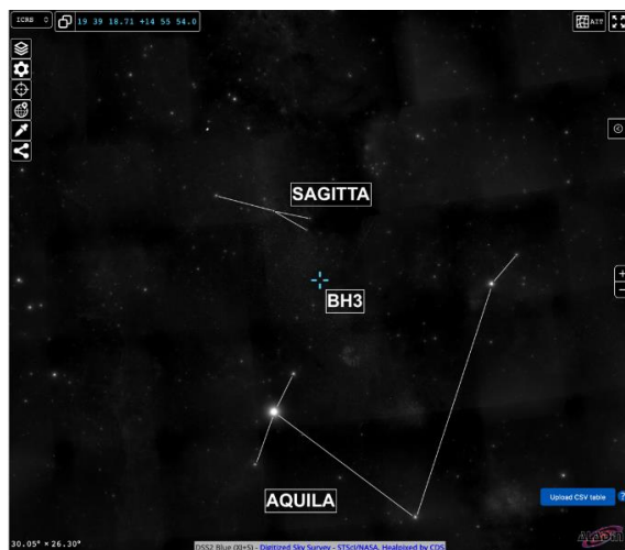
Figure 2: Localisation du trou noir BH3 (croix bleue) par rapport aux constellations de la Flèche et de l'Aigle (Image générée par Aladin Lite).
