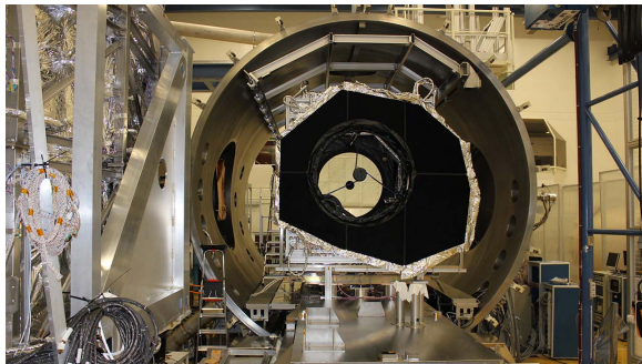
Le télescope spatial Euclid, de passage au Centre Spatial de Liège pour des essais sous vide, en 2021.
